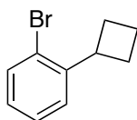
1-bromo-2-cyclobutylbenzene
