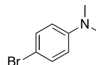
para-(Me 2 N)BrC 6 H 4
