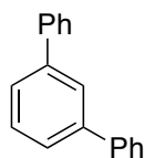
1,3-diphenylbenzene
